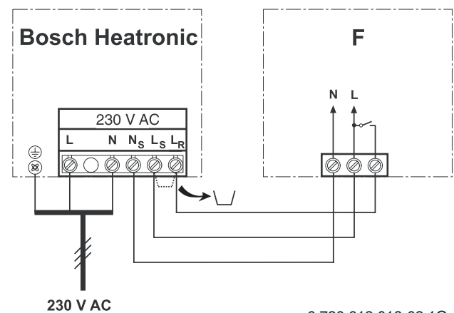
Fig. 14 Conexión con un termostato ON/OFF TR..F (230 V AC)
